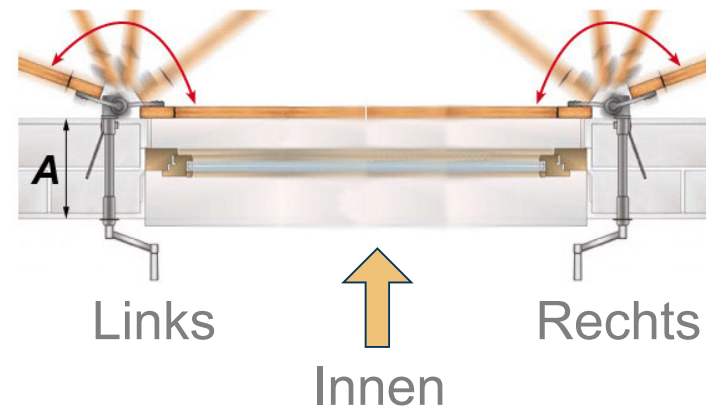
2F/1R1L Zweiflügelig Fenster / 1 Einfachflügel links, 1 Einfachflügel rechts
